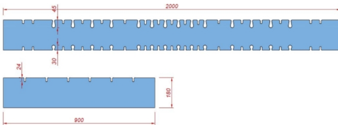
HR ULTRA nagy tömörsűrűségű hideghab matrac vágási metszete
